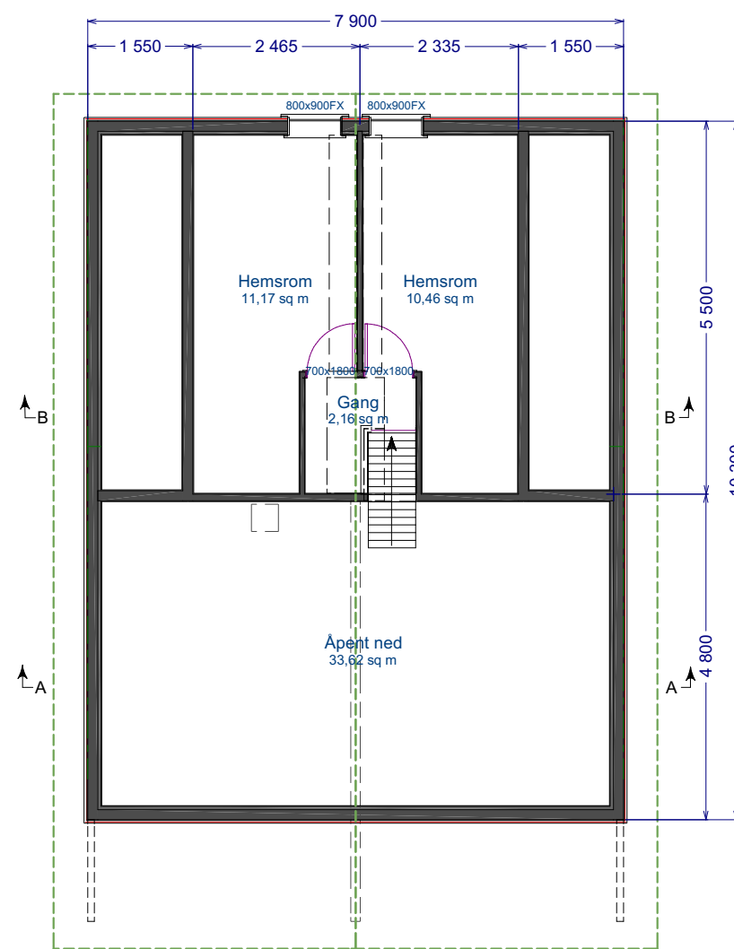
Plantegning loftsetasje
