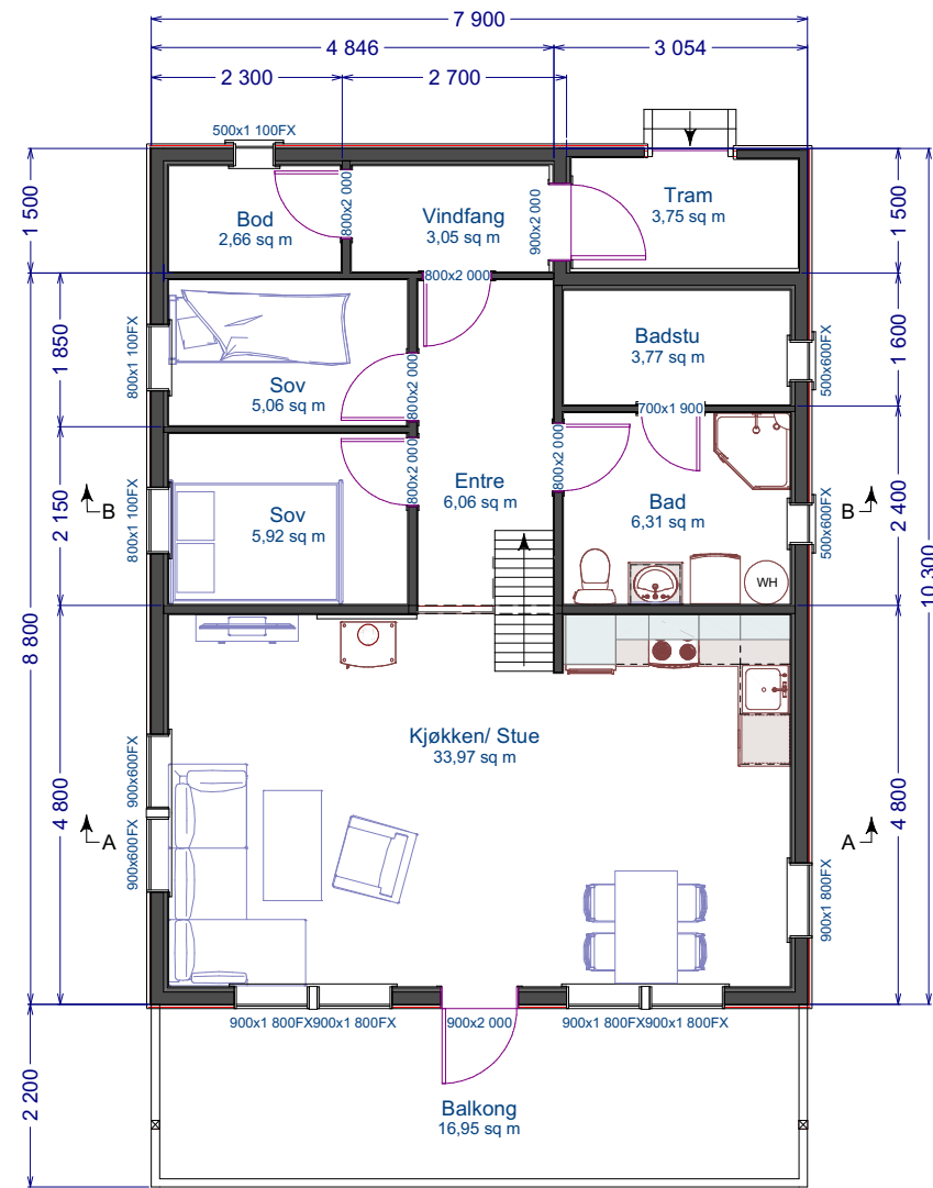
Plantegning 1. etasje
